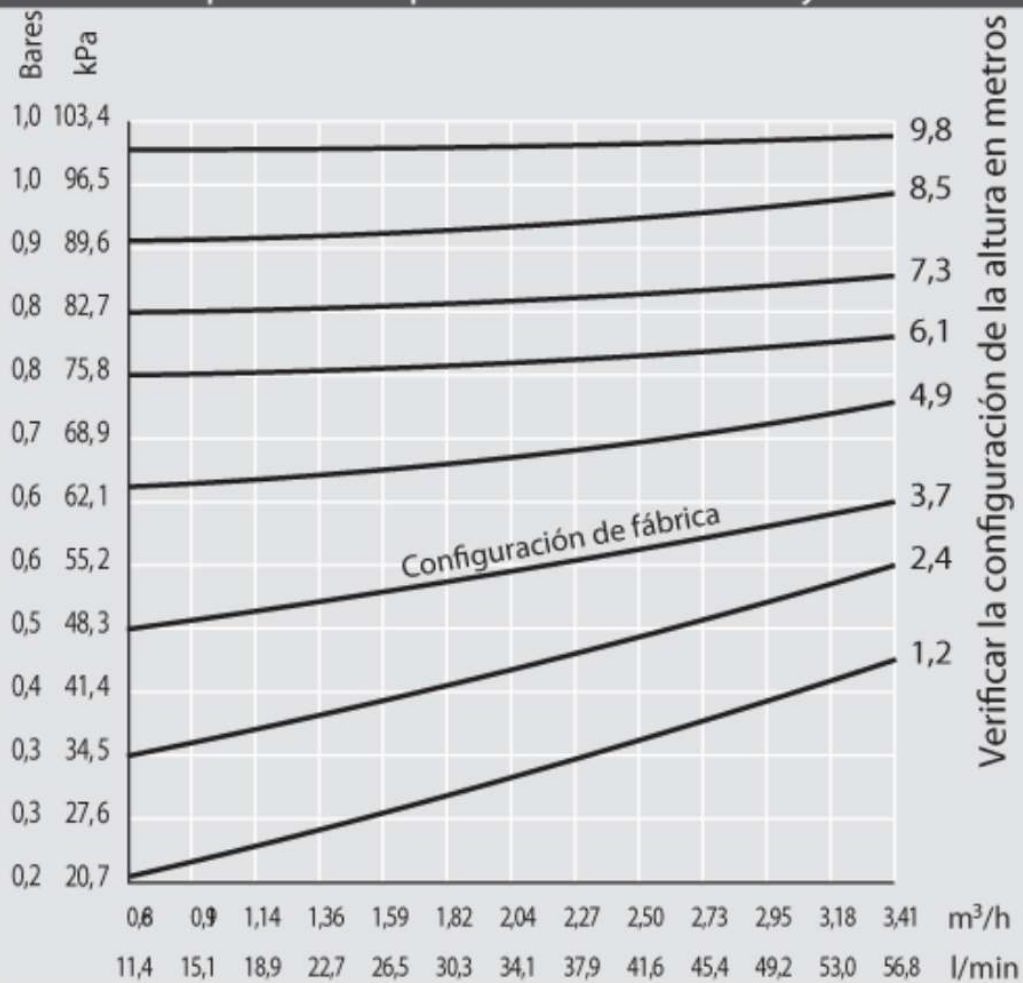
Gráfico de pérdida de presión HCV en bares y kPa
