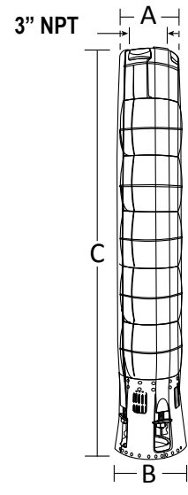
Acoplamiento NEMA 8"
