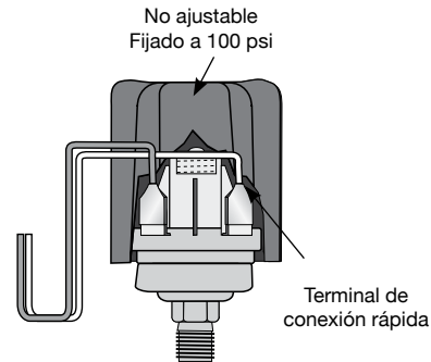
Figura 5B: Interruptor para presión de corte
