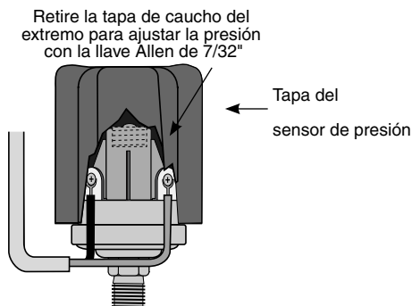
Figura 5A: Sensor de presión
